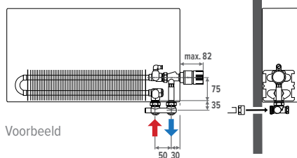
AANSLUITING RECHTS
